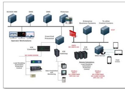
자동화 시스템 아키텍처
